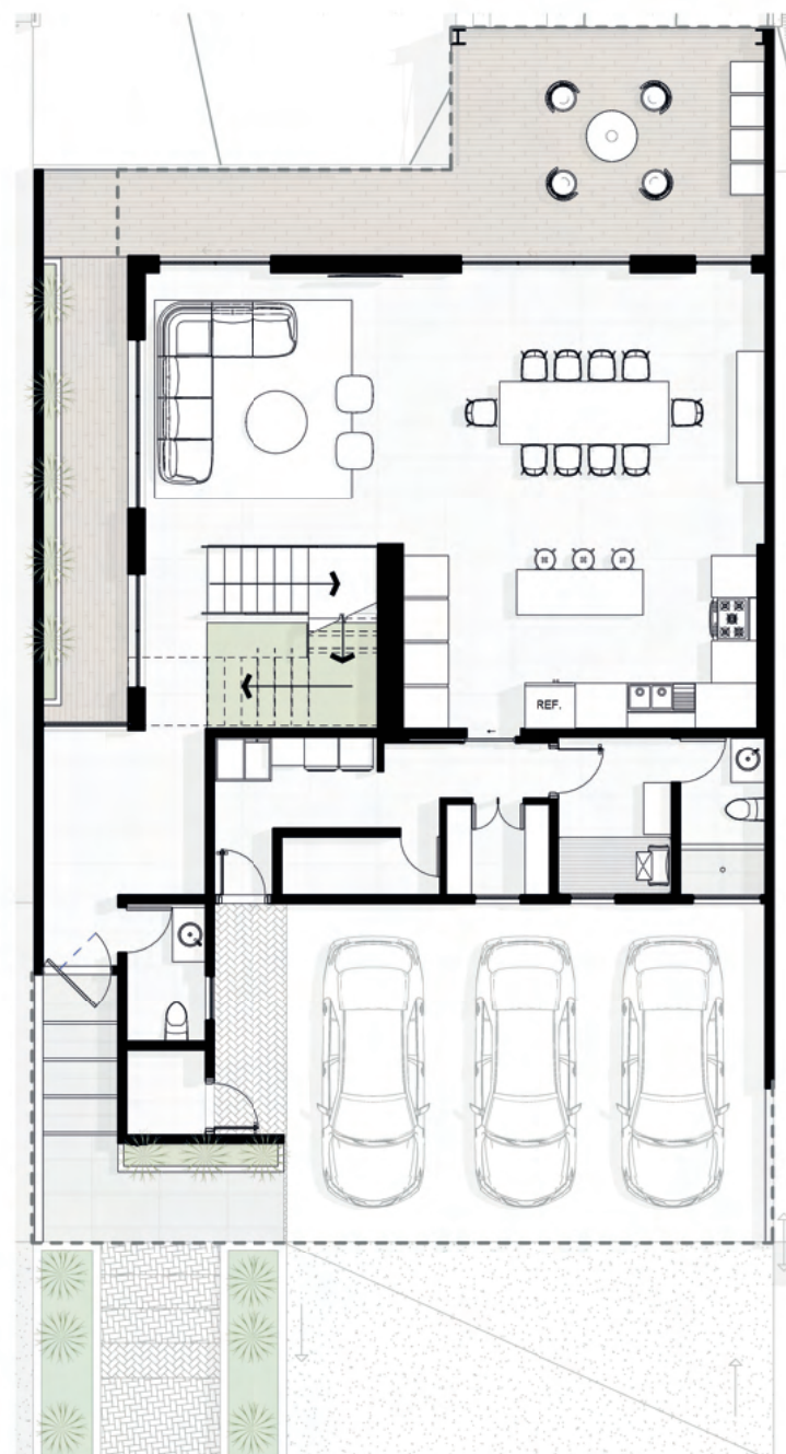
Primer Nivel Planta de Arquitectura
