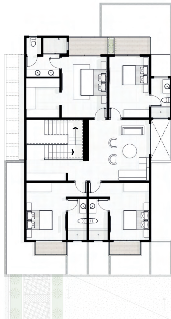
Segundo Nivel Planta de Arquitectura
